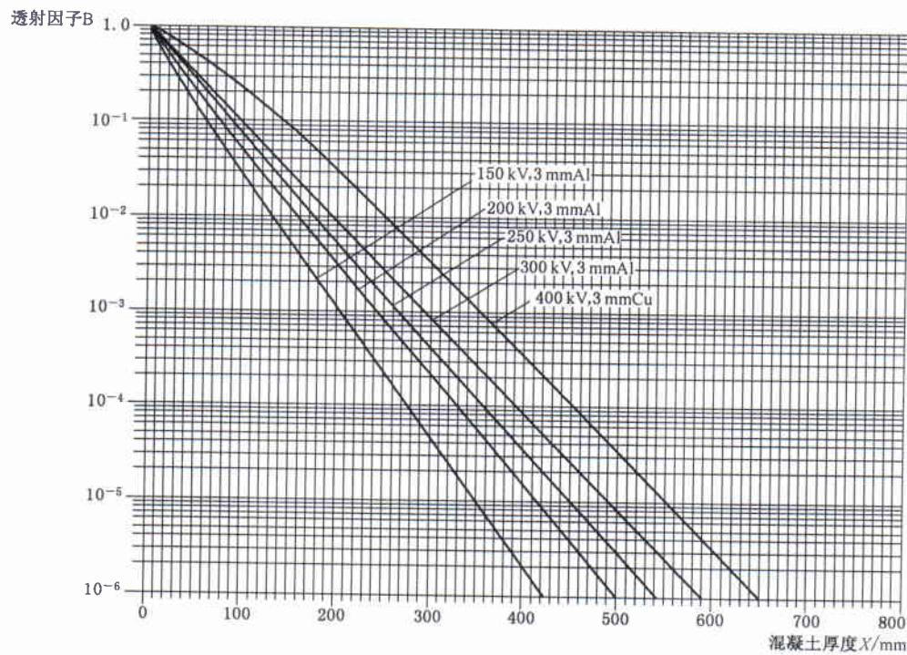
图 B.2 X 射线穿过混凝土的透射
